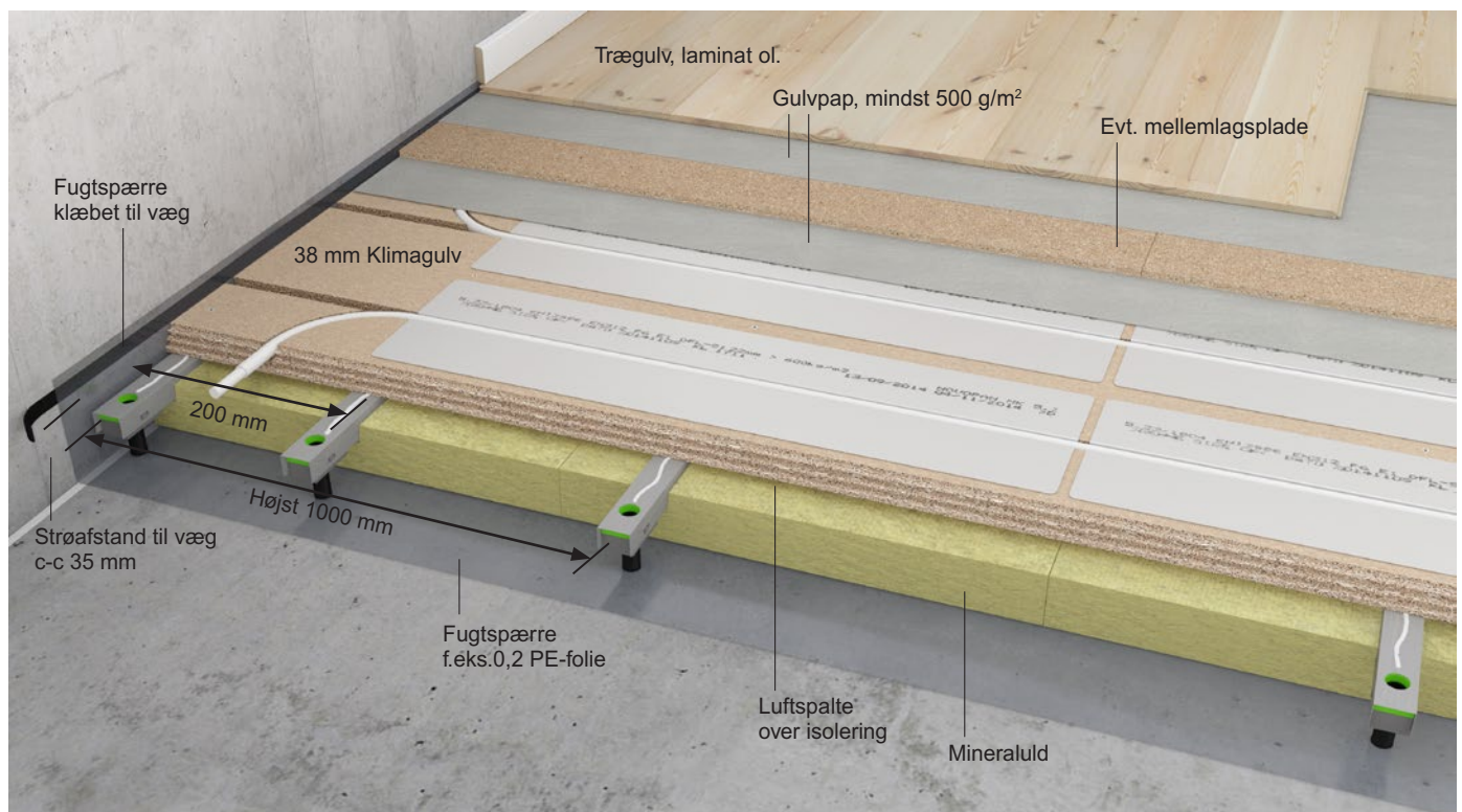
Figur 1 38 mm Novopan Klimagulv med fræsede vendespor udført efter lægning af gulvpladerne. Vendespor skal understøttes af en ekstra stålstrø 200 mm fra væg.
